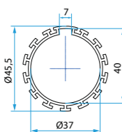
A3505_0510 Adattatori tubo Tondo 40 sp. 1,5 mm con dente
