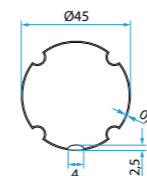
A3505_0504 Adattatori tubo ZF 45
