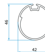
A3505_0508 Adattatori tubo Ovale 42X46
