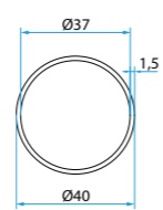
A3505_0511 Adattatori tubo Tondo 40 sp. 1,5 mm
