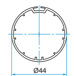
A3505_0515 Adattatori tubo Tondo Filtersun 44
